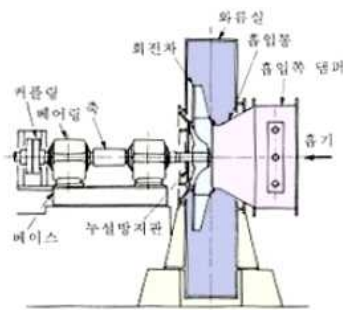
그림 1. 원심식 송풍기 구성
