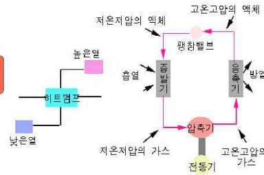
히트펌프 시스템 구성요소 및 동작원리
