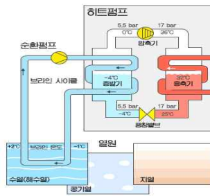
히트펌프 시스템 구성요소 및 동작원리
